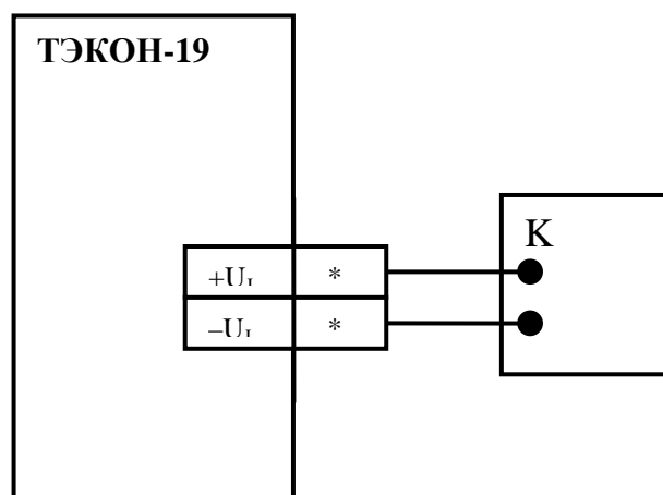
Рисунок 6.2 - Схема подключения средств поверки при проведении поверки ИК силы тока. K – калибратор тока, * – номера контактов по таблице 3.1
