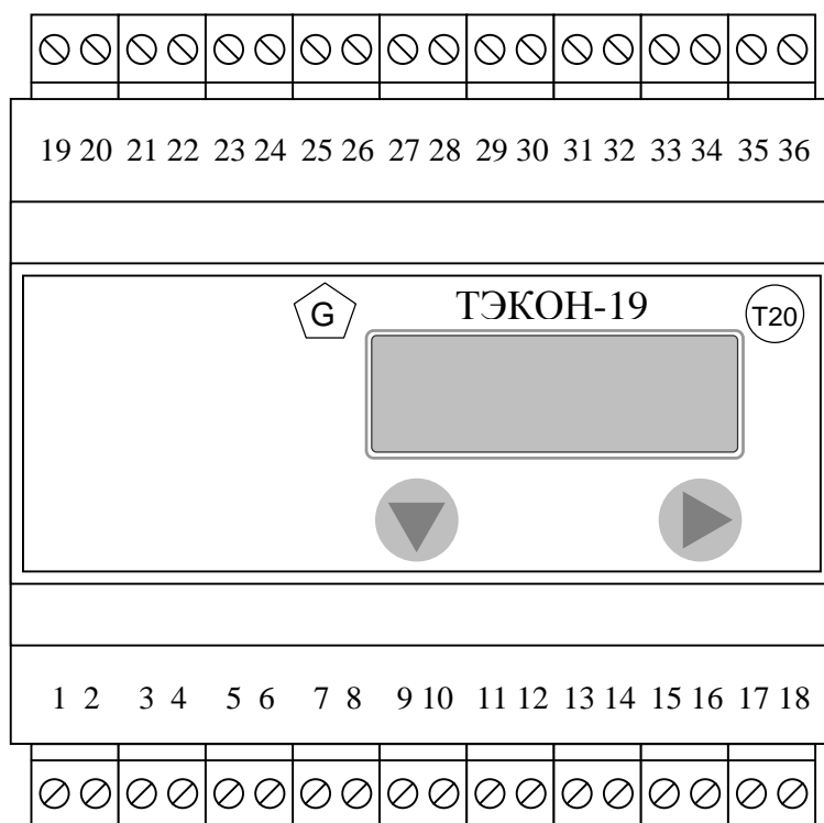
Рисунок 2.1 – Внешний вид передней панели и нумерация клемм ТЭКОH-19 для различных исполнений:
