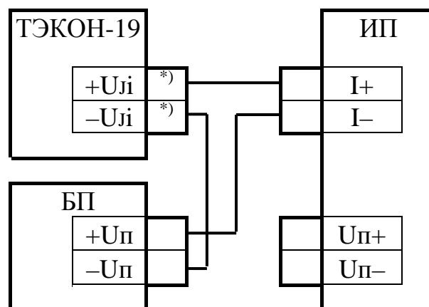
б) двухпроводная
