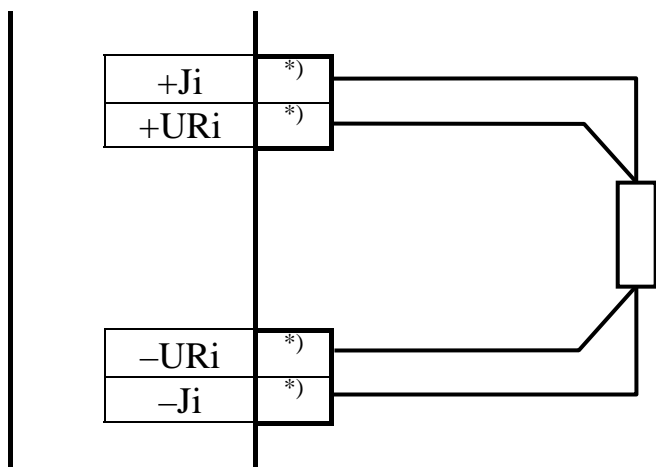
а) Схема подключения
