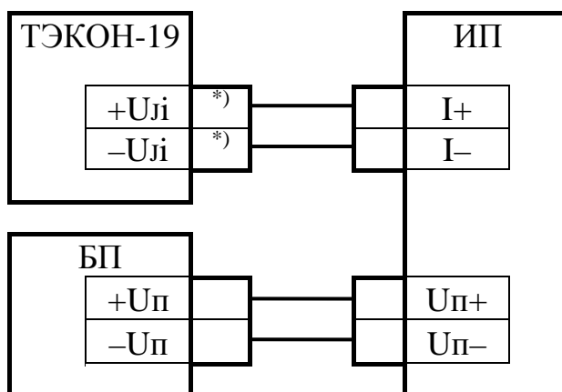
а) четырехпроводная
